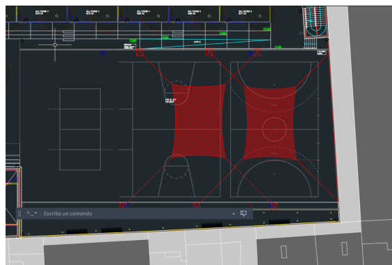
Projecte inicial de veles sobre la pista.
